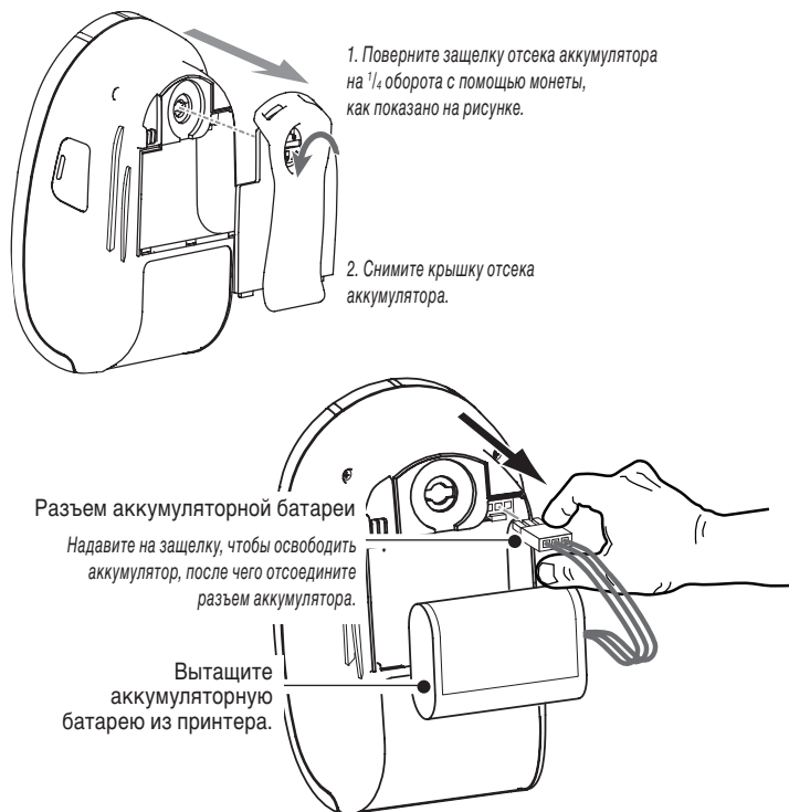
Рисунок 2.2. Извлечение аккумулятора.
