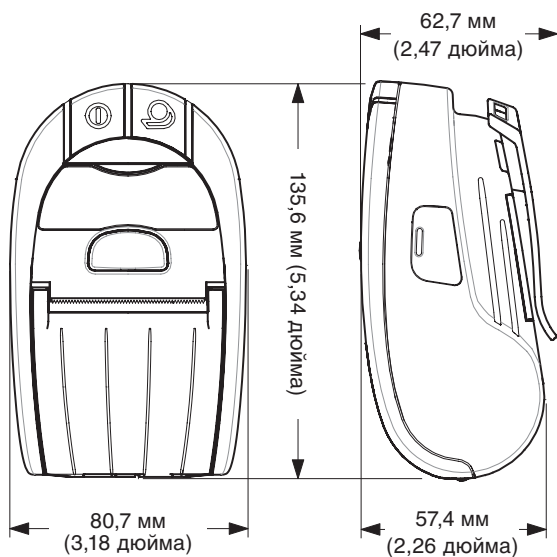
Рисунок 18. Габариты принтера MZ 220.
