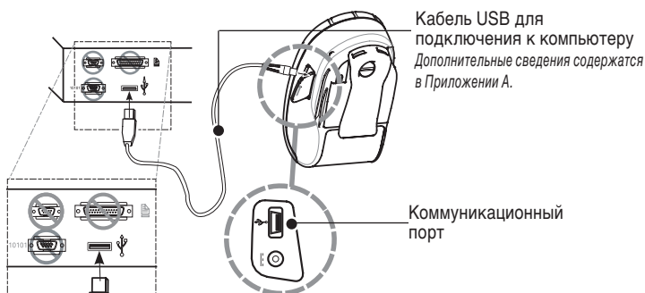
Рисунок 11. Подключение к ПК.
