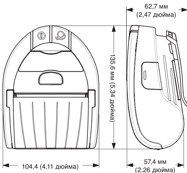
Рисунок 19. Габариты принтера MZ 320.
